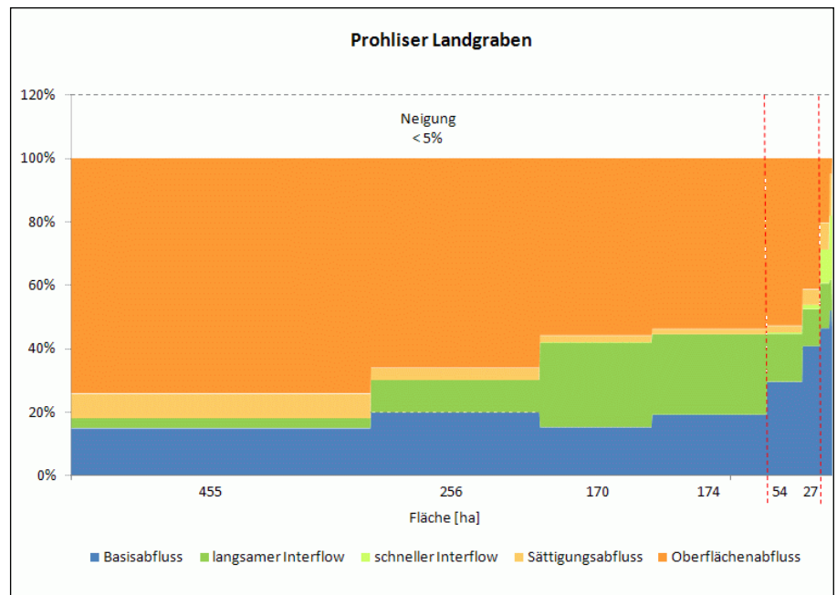
Abb. 24: Relative Anteile der Abflussbildung im Einzugsgebiet bei mittlerer Bodenvorfeuchte (die der Grafik zugrundeliegenden Daten wurden im Jahr 2008 für die aktuelle Flächennutzung mittels WBS FLAB ermittelt)
