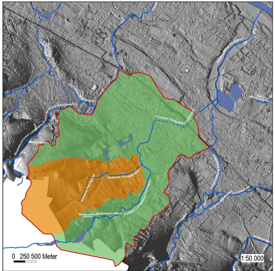
Abb. 17: Einzugsgebiet des Prohliser Landgrabens/Geberbaches innerhalb von Dresden
