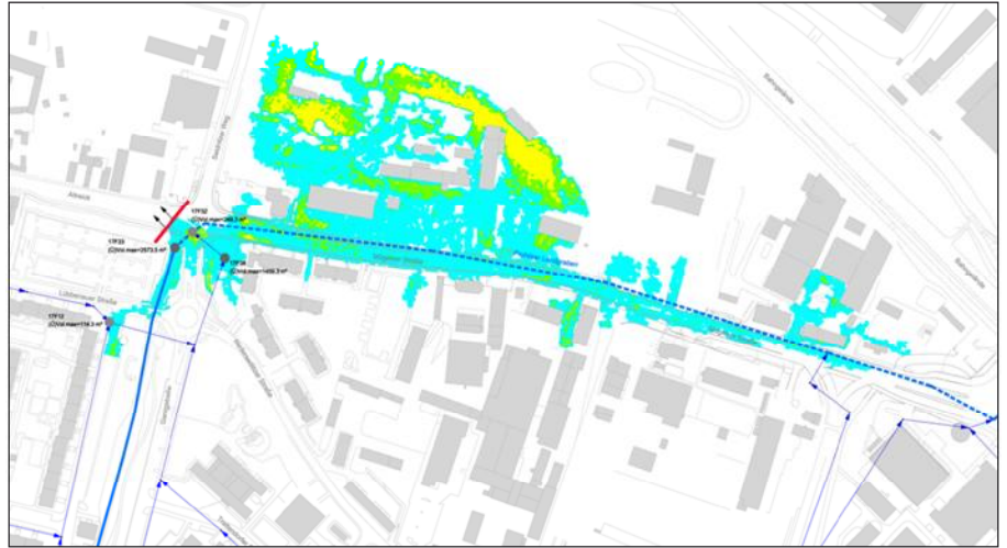
Abb. 32: Überflutungsgefährdete Bereiche durch Überstau am Einlauf in die Verrohrung Mügelter Straße (türkis: Überflutungshöhe kleiner 10 cm, gelb: Überflutungshöhe 20 bis 50 cm)
