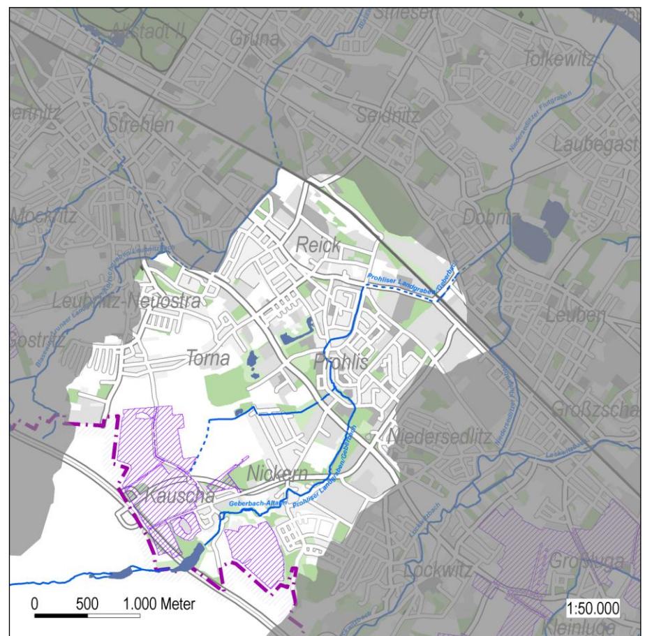
Abb. 26: Gebiete mit nutzungsbedingt erhöhtem Oberflächenabfluss an Prohliser Landgraben/Geberbach und Nickerner Abzugsgraben
