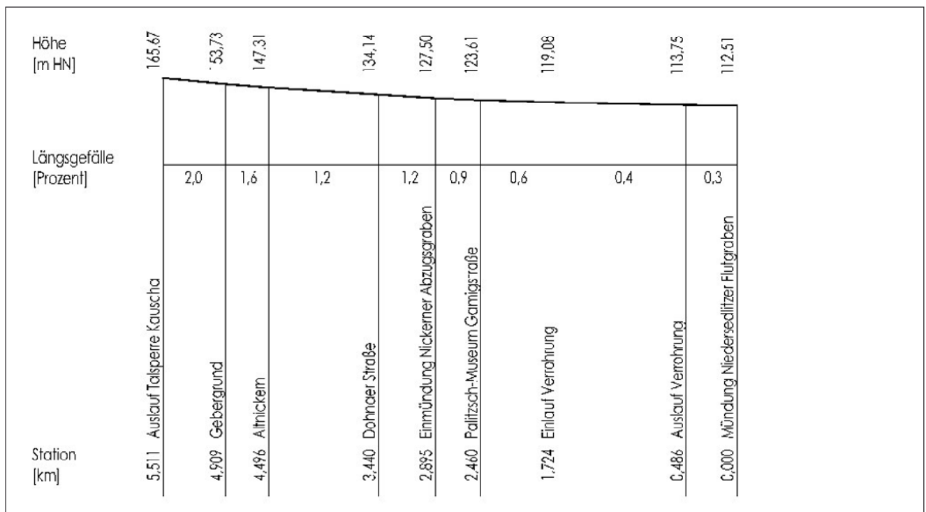
Abb. 12: Morphologischer Gewässerlängsschnitt Prohliser Landgraben/Geberbach
