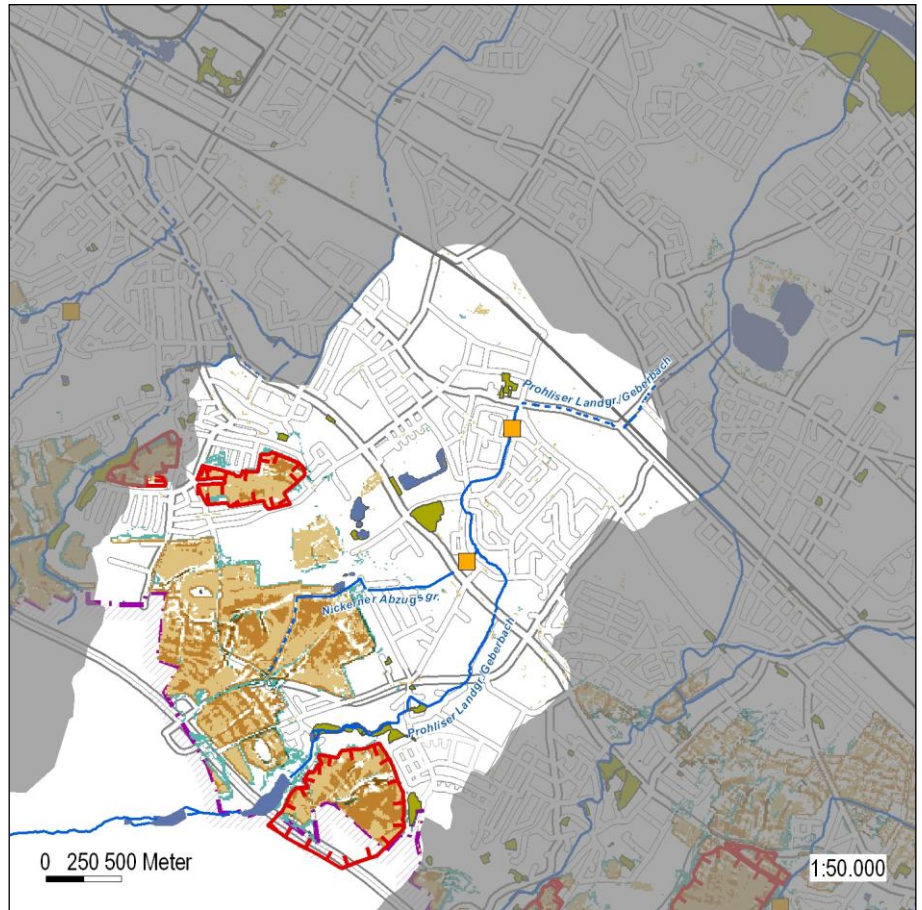
Abb. 27: Erosionsgefährdete Flächen (beige/braun) und Deposition (türkis) im Einzugsgebiet des Prohliser Landgrabens/Geberbaches und des Nickerner Abzugsgrabens
