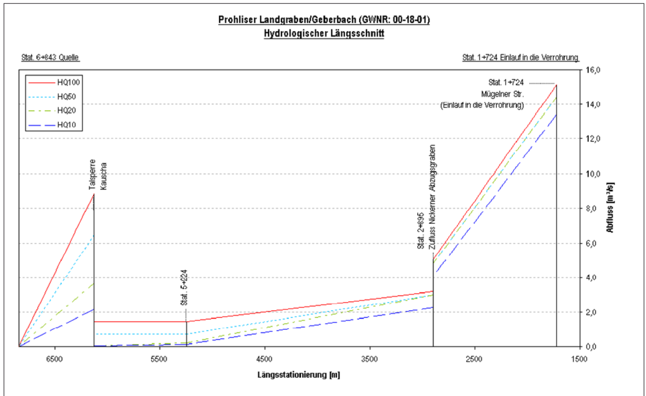
Abb. 16: Hydrologischer Gewässerlängsschnitt
